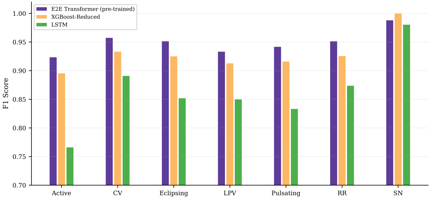
Per-Class F1 Scores
